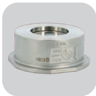
CLAPET DE RETENU A DISQUE 386
